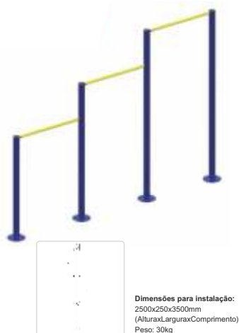
BARRA FIXA Código APA0129
