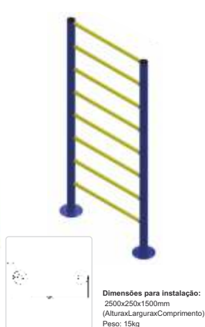
MULTI-ALONGADOR Código APA0123
