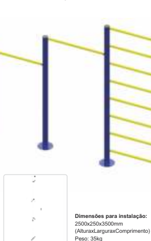
JOGO DE BARRAS COM ESPALDAR Código APA0102
